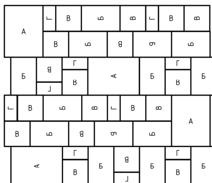
Раскладка типовая (линейная)
