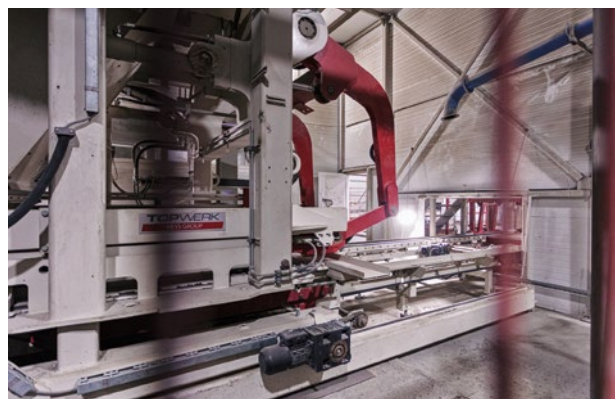
Мощный вибропресс HESS Multimat-2000
